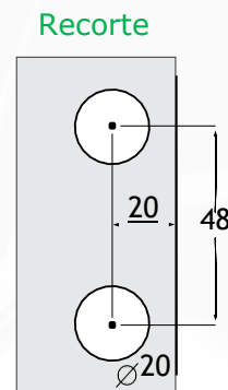
Ref.: 3214-M Mini fechadura sem tambor externo para janela de bater
