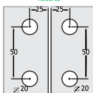
Ref.: 1129-E Dobradiça ESQUERDA dupla automática vidro/vidro
