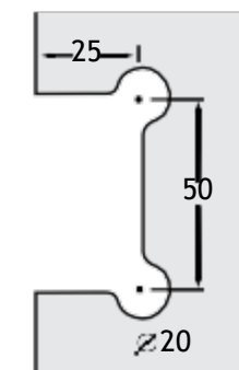
Ref.: 1131 Dobradiça para porta de bater com ponto de giro deslocado a 30mm
