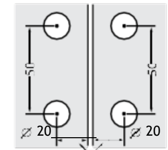
Ref.: 1129-D-ÂNG Dobradiça DIREITA dupla automática vidro/vidro para ângulo
