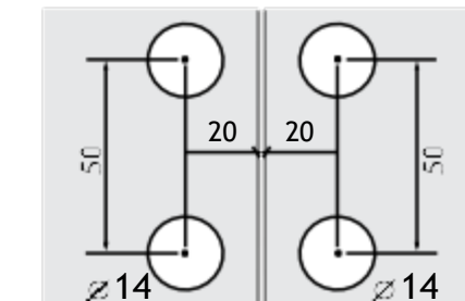
Ref.: 1570-PR BATE-FECHA - Fecho de pressão para vidro laminado
