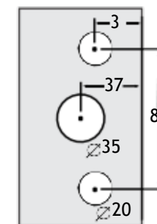
Ref.: 3536-90° Contra fechadura para fech. 3532 c/ fechamento em 90°
