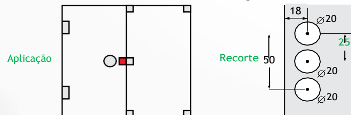
Ref.: 1529-FC-D e 1529-FC-E Fechadura para porta de box de bater direita / esquerda vidro / vidro - montagem com a 3211-M Vidro / alvenaria - montagem com a 3230-M
