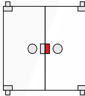
Ref.: 1504-A Espelho com batente para fechadura 1520
