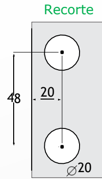
Ref.: 3212-M Mini contra fechadura sem batente para fech. 3214-M
