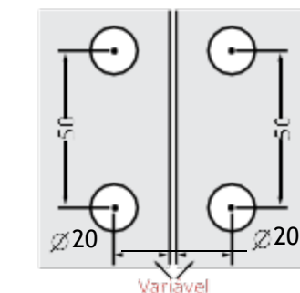
Ref.: 1130 Suporte para basculante e pivotante com pino
