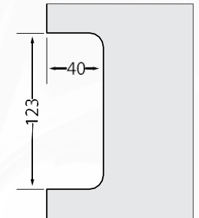
Ref.: 1510 JE Fechadura bico de papagaio ESQUERDA para janela
