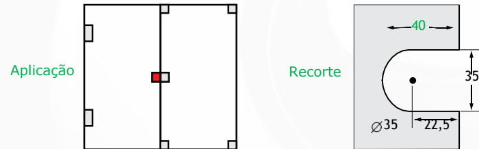
Ref.: 1529-FC-D e 1529-FC-E Fechadura para porta de box de bater direita / esquerda vidro / vidro - montagem com a 3211-M Vidro / alvenaria - montagem com a 3230-M
