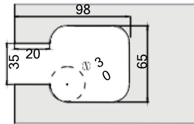
Ref.: 1128-C Dobradiça horizontal vidro/vidro com ponto de giro de 65mm
