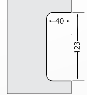
Ref.: 1510 JD Fechadura bico de papagaio DIREITA para janela
