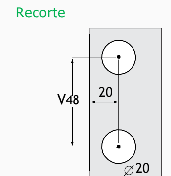
Ref.: 3536-M Mini contra fechadura para fechadura 3532-M
