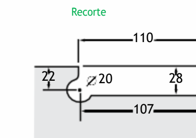
Ref.: 1105 Dobradiça esquerda superior excêntrica
