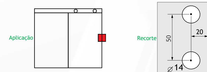
Ref.: 1710-TQ Conjunto mão de amigo
