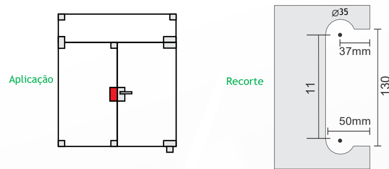
Ref.: 1509-TQ Espelho para 1507-TQ
