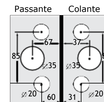
Ref.: 3536-PR Contra fechadura de pressão para fechadura 3532-PR
