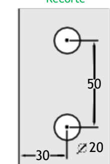
Ref.: 1131 Dobradiça para porta de bater com ponto de giro deslocado a 30mm
