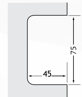
Ref.: 1520-T (tetra) Fechadura para porta de bater com chave tetra
