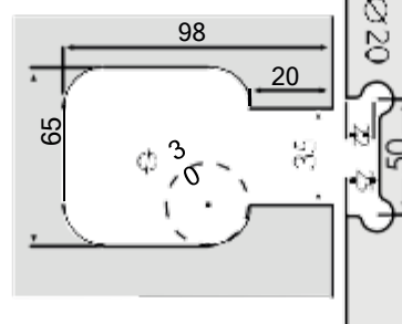
Ref.: 1129-D Dobradiça DIREITA dupla automática vidro/vidro
