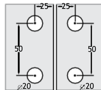
Ref.: 1129-E Dobradiça ESQUERDA dupla automática vidro/vidro
