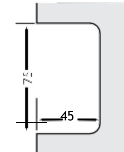
Ref.: 1531 Contra Fechadura com batente para fechadura: 1520/1520-T
